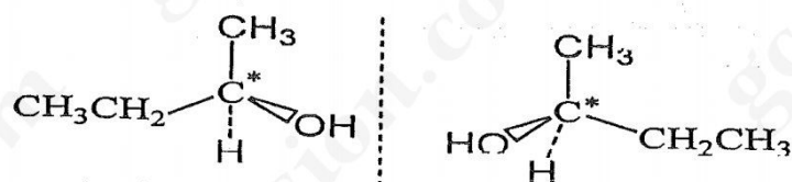
Enantiomers
