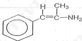
cis-1-phenylprop-1-en-2-amine
